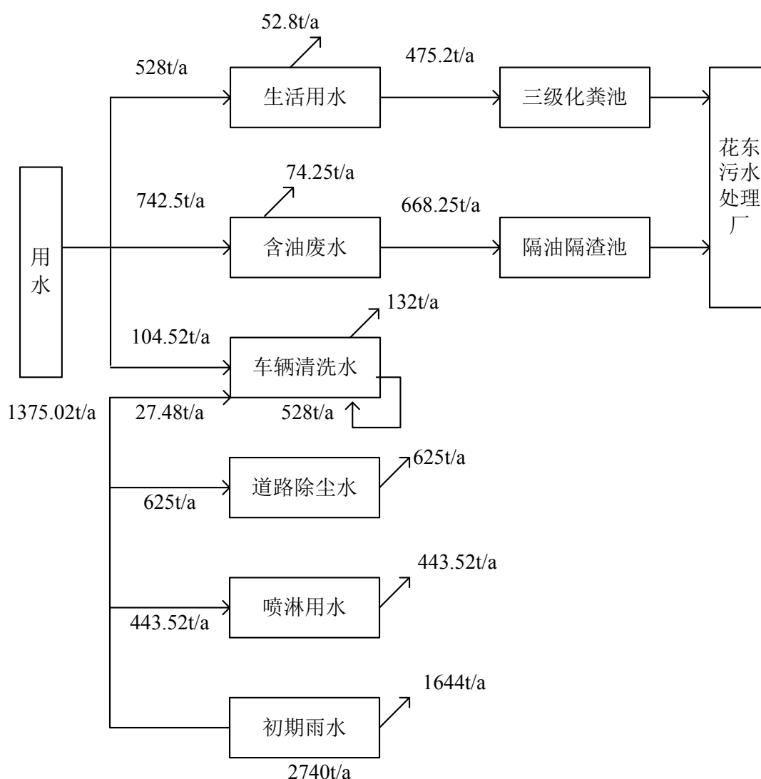
图5-3 项目水平衡图
